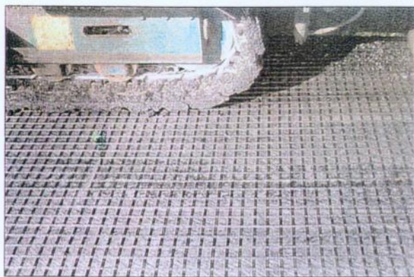
Bild 3: Befahren von HaTelit C 40/17 mit Kettenfertiger
