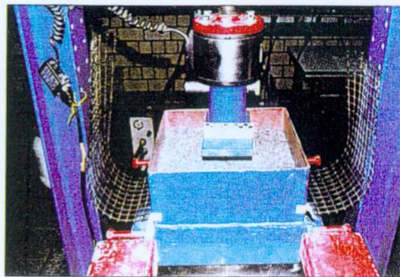
Bild 5: Versuchsaufbau
